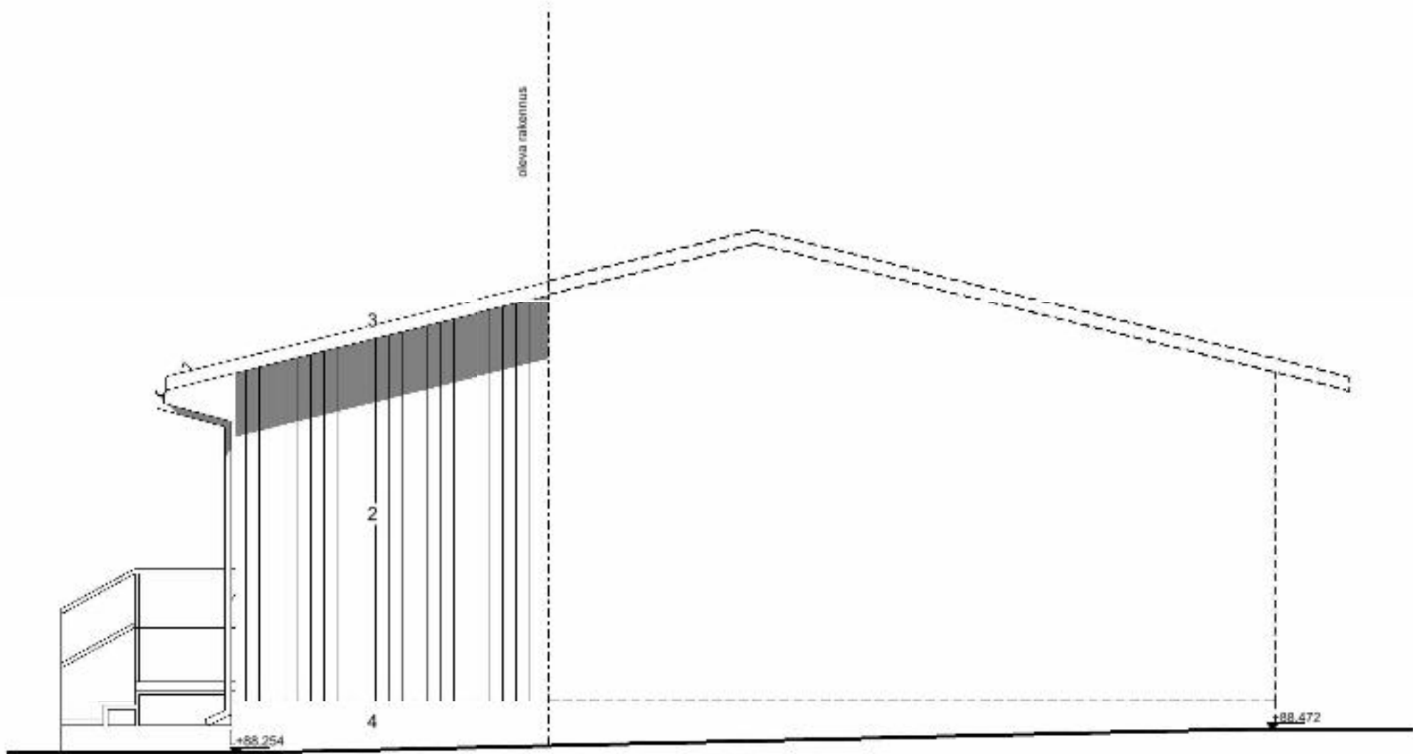
Julkisivu lounaaseen
